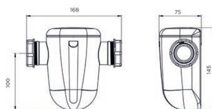
Dimensiones (mm)
