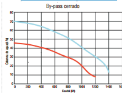
Gráfica (caudal/presión) VICTRIX
